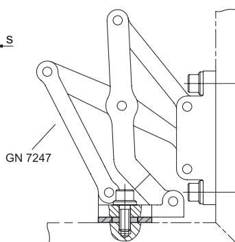
Montagebeispiel
